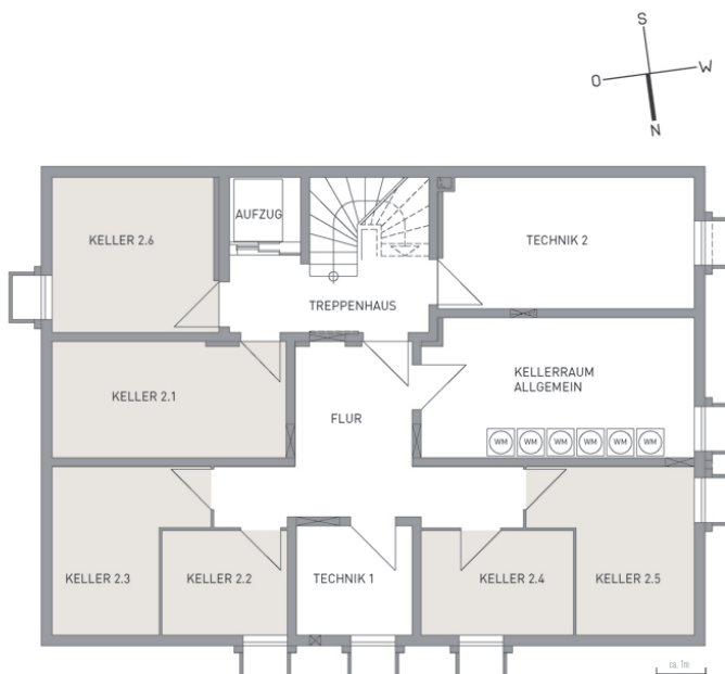
Haus 2 UG
